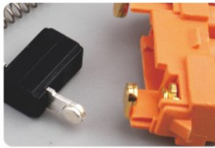
加粗触点,通过电流更大 Big Contact
