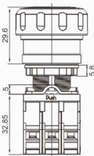
M1急停(塑料红色头部)
