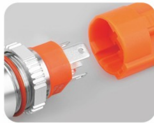
可配专用插件 Connector
