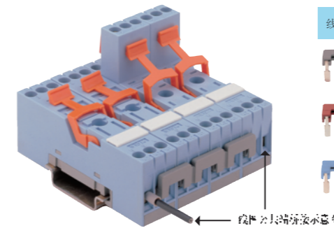
线圈末端的插入式桥接片B20
