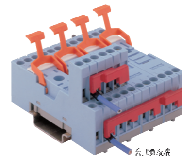
负载末端的插入式桥接片
