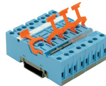
桥接片S10-BB, 可用于S10底座的线圈端A2或负载端
