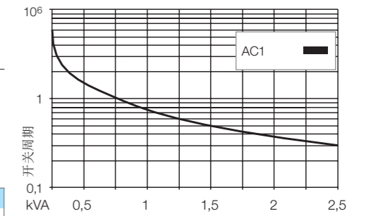
示意图2 最大直流负载
